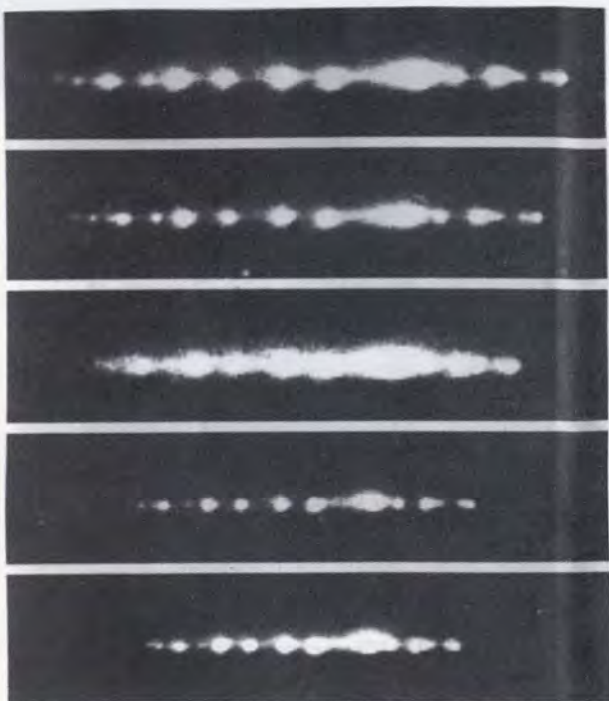
Shoemaker-Levy 9 kometaren zatiketa. Goitik behera: 1993eko martxoak 27, apirilak 15, maiatzak 21, ekainak 12 eta uztailak 17.
